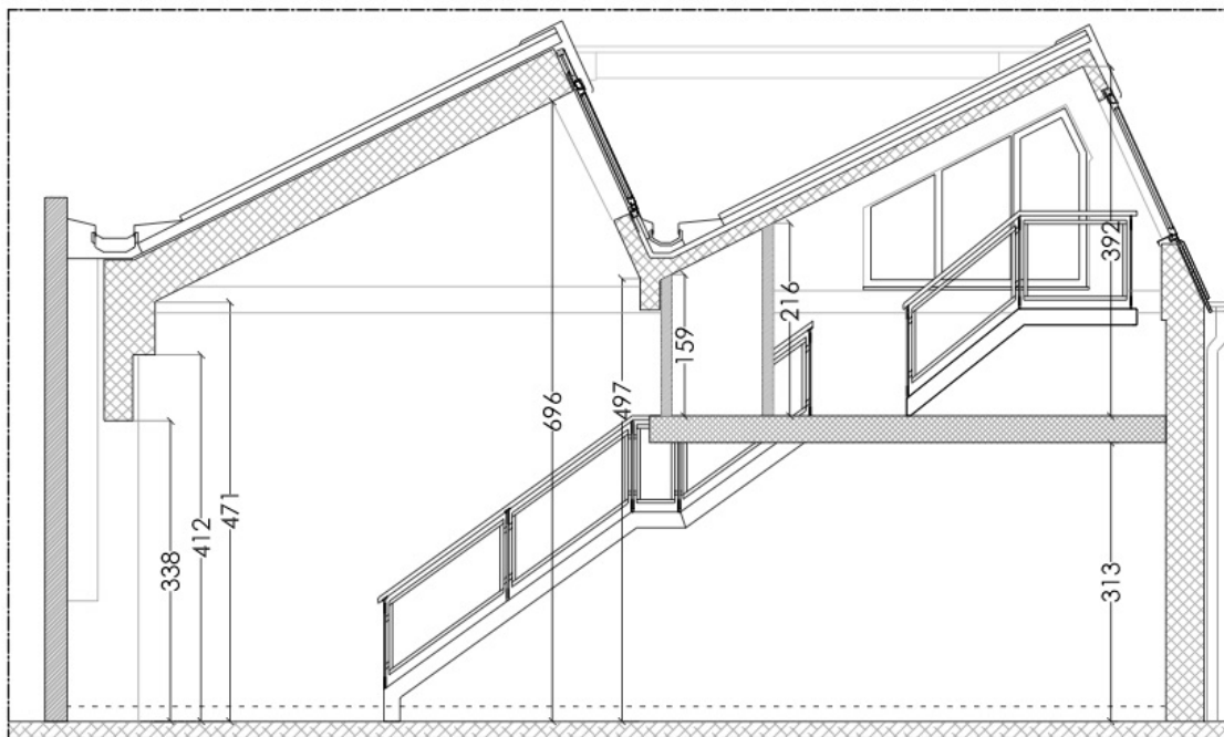
Stato di Fatto - Sezione A scala 1:100
