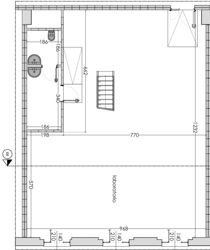
Stato di Fatto - Piano Terra scala 1:100
