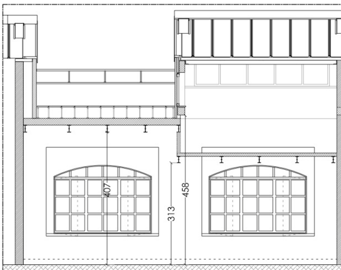
Stato di Fatto - Sezione B scala 1:100
