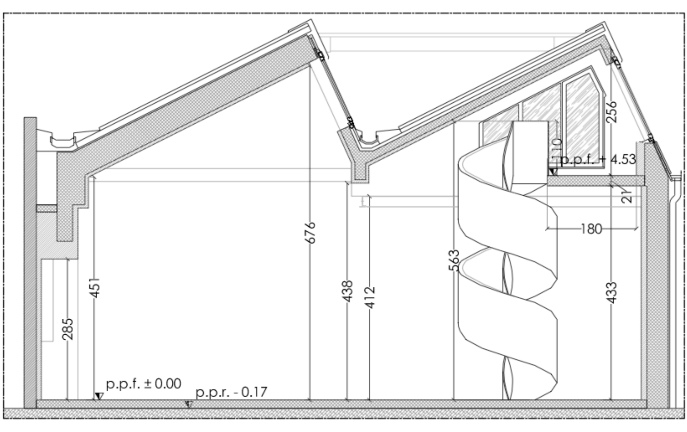
Stato di Progetto - Sezione A scala 1:100
