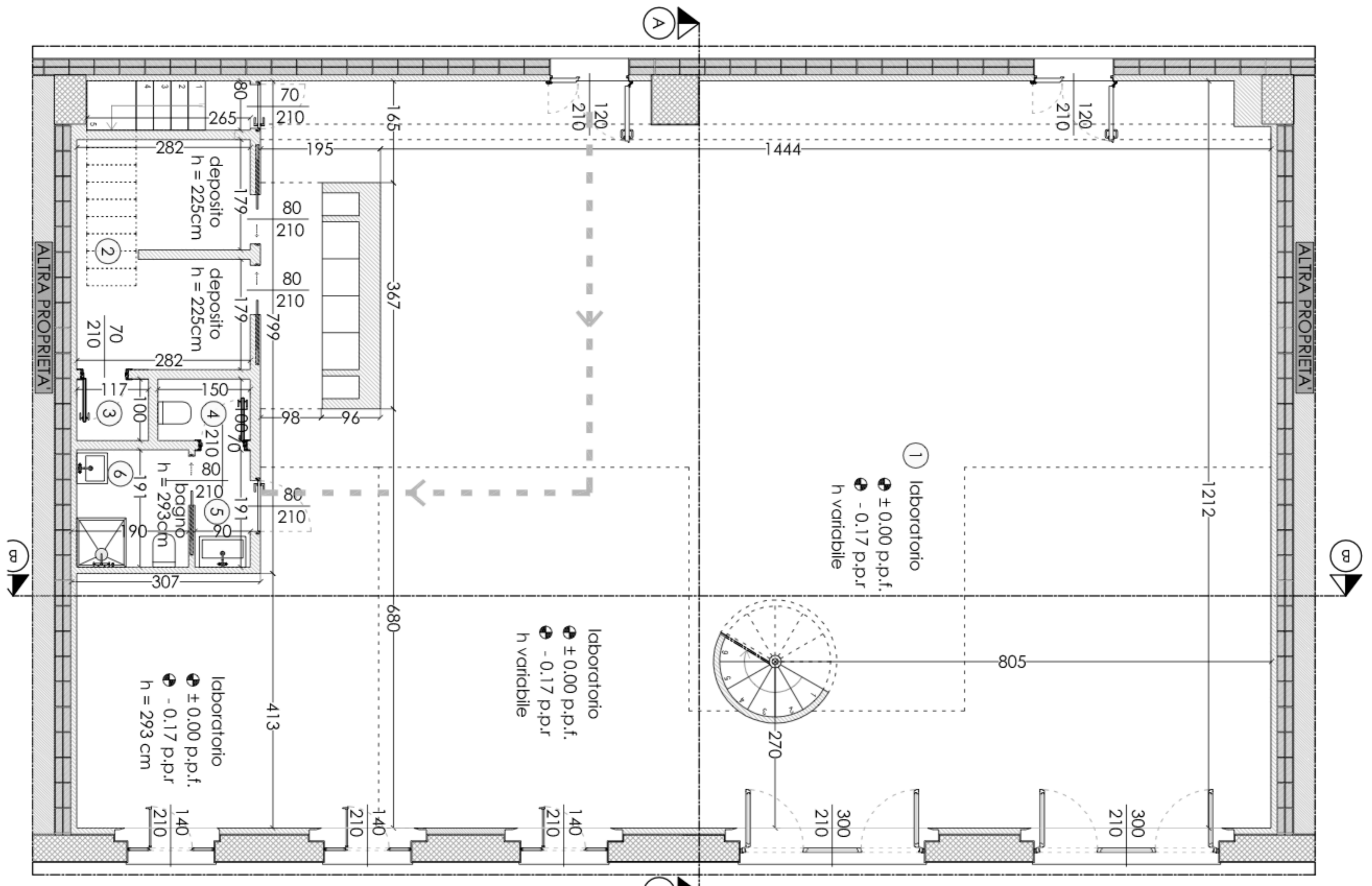
Stato di Progetto - Piano Terra scala 1:100
