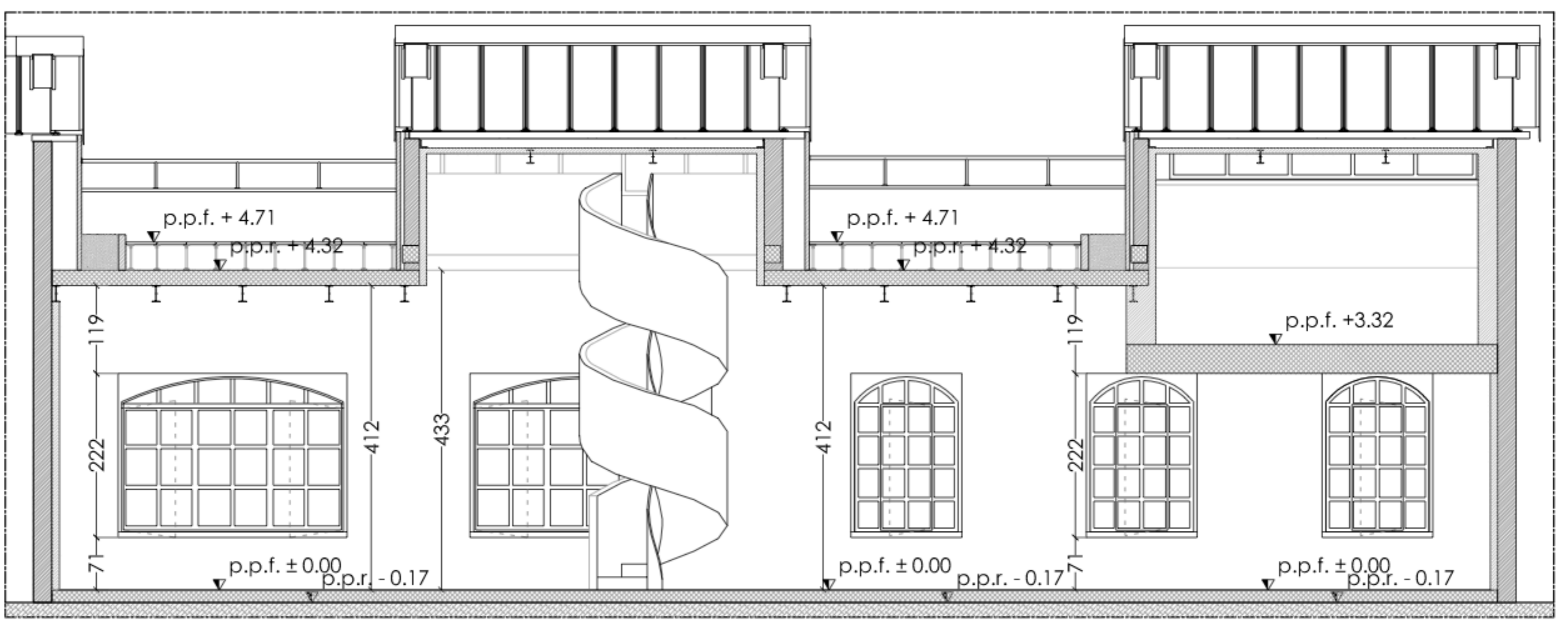
Stato di Progetto - Sezione B scala 1:100
