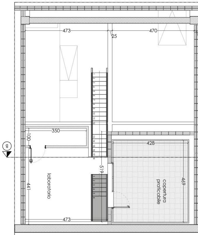
Stato di Fatto - Piano Primo scala 1:100
