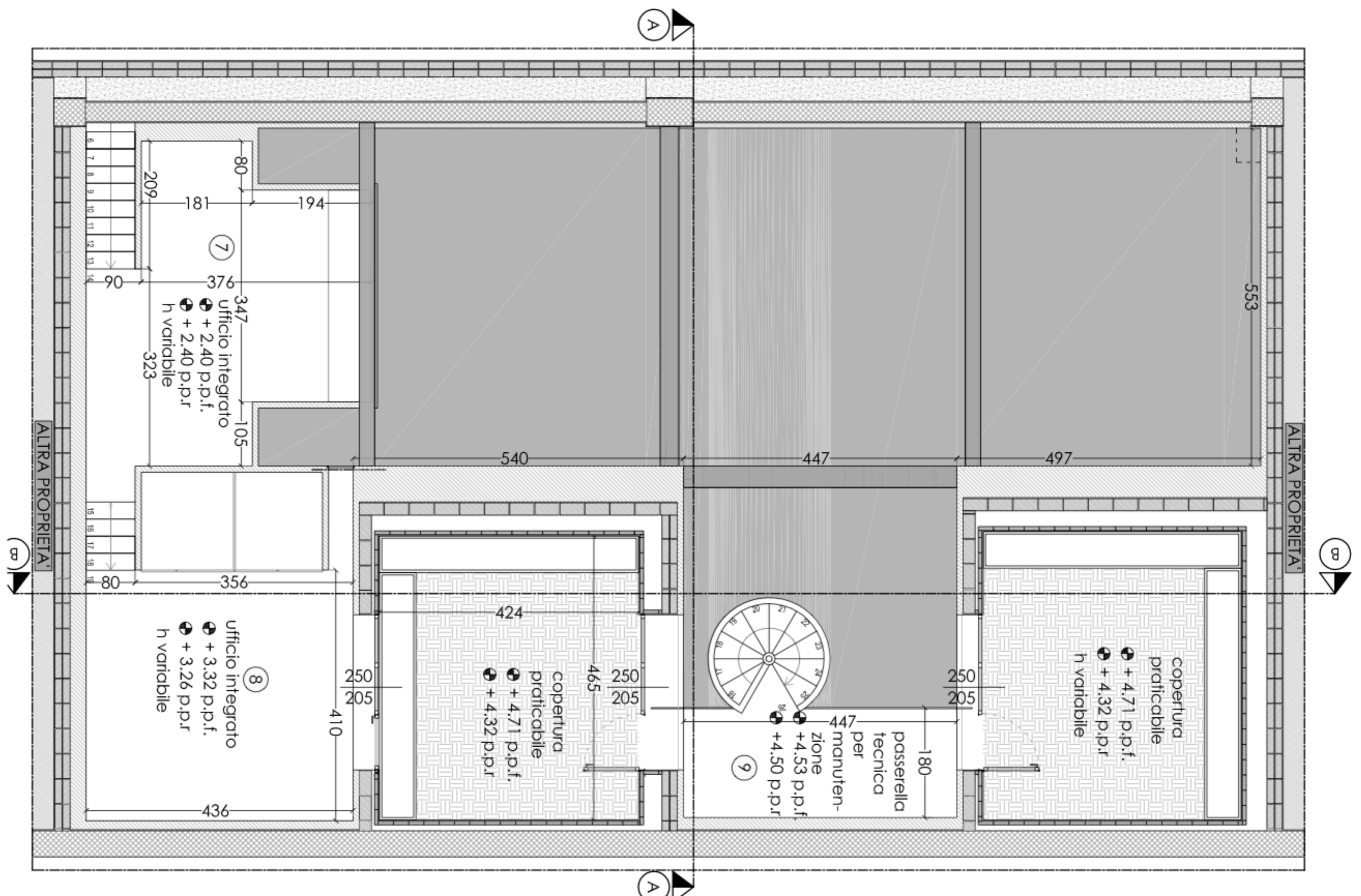
Stato di Progetto - Piano Primo scala 1:100
